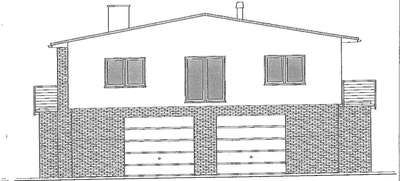
Sudansicht
