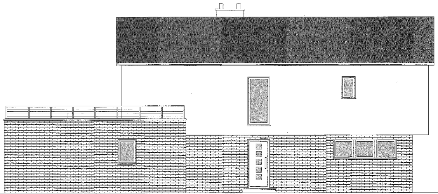
Westansicht
