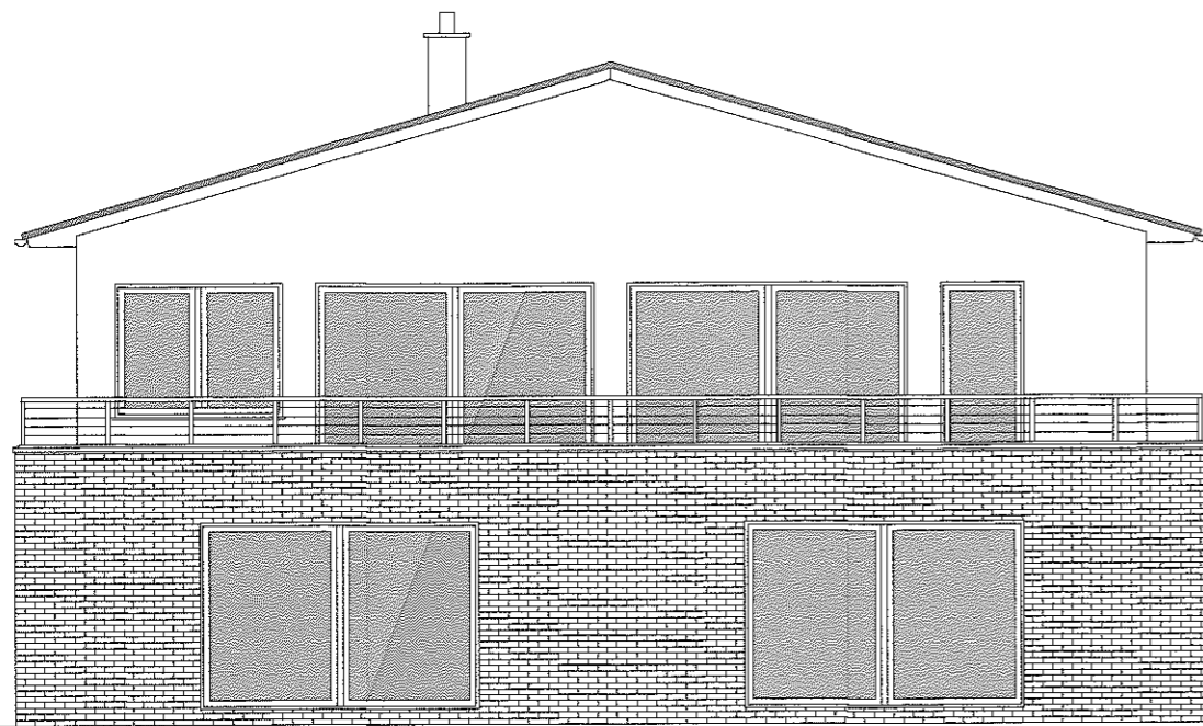
Gartenansicht
