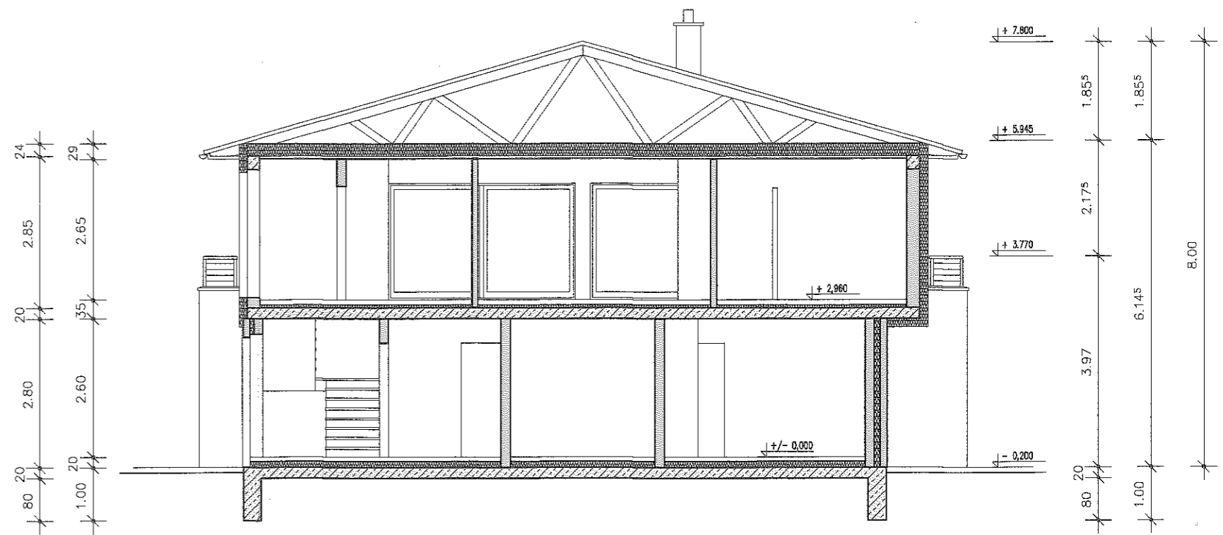
Schnitt A-A
